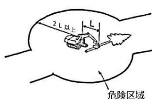
造材作業
